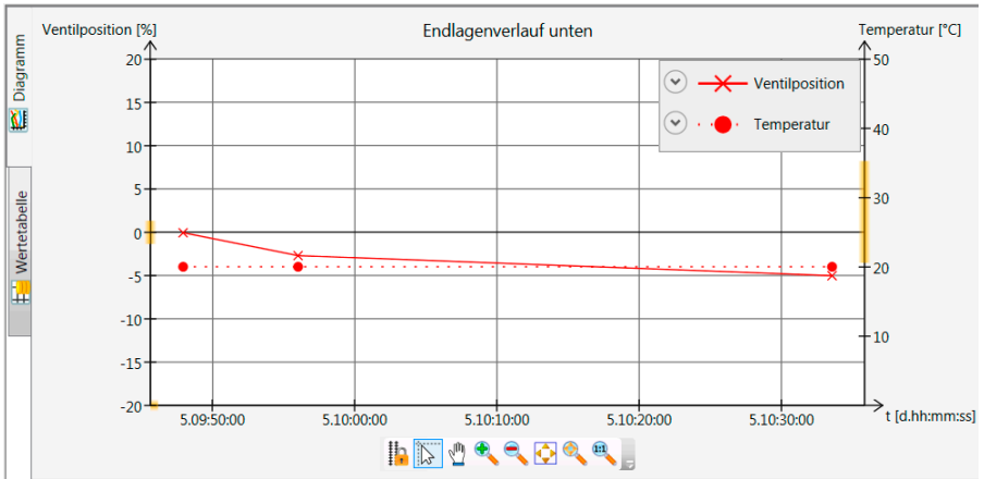
Bild 7: > Diagnose/Wartung > Beobachtung > Endlagenverlauf > Unterer Endlagenverlauf
