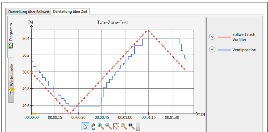
Bild 17: > Diagnose/Wartung > Testfunktionen > Tote Zone > Darstellung über Zeit
