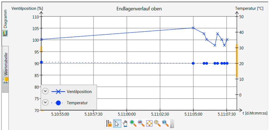
Bild 8: > Diagnose/Wartung > Beobachtung > Endlagenverlauf > Oberer Endlagenverlauf
