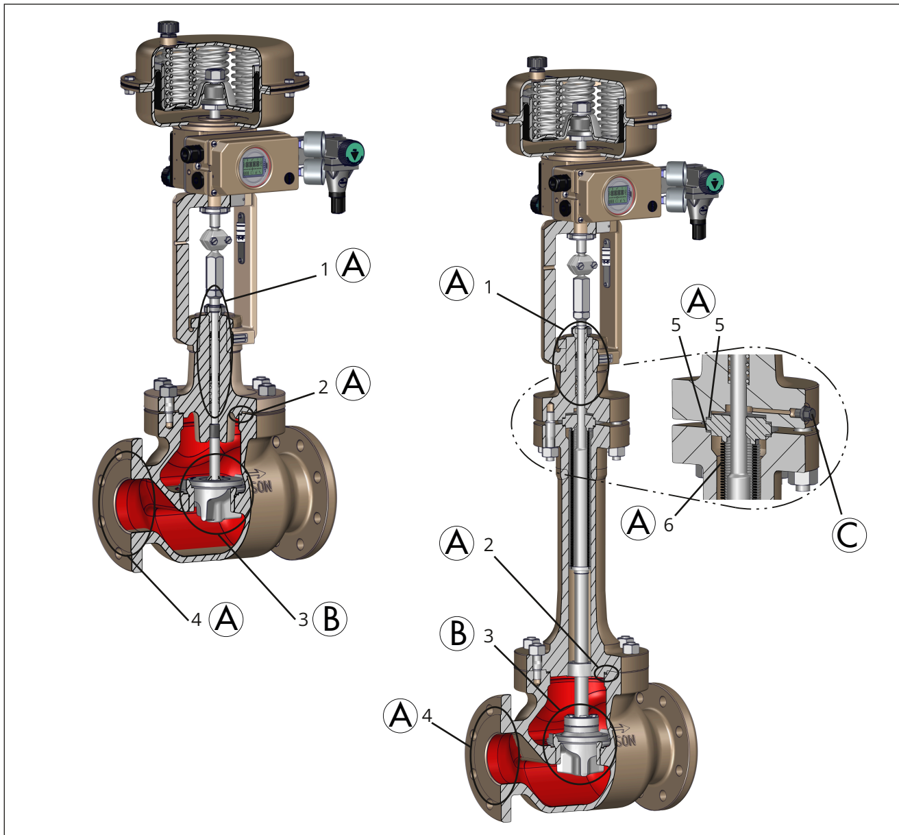
Bild 32: Darstellung möglicher Leckagezonen am Stellventil (Beispieldarstellungen: links Ausführung mit Standardoberteil - rechts Ausführung mit Balgteil, stellvertretend auch für Ausführungen mit Isolierteil oder Zwischenstück).
