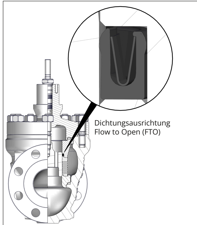
Bild 35: Ausrichtung der Dichtung (45) am Käfig bei Durchflussrichtung FTO (Flow to Open)
