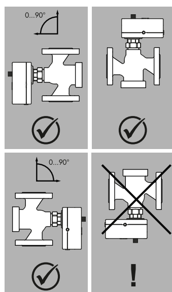
Bild 4: Einbaulage
